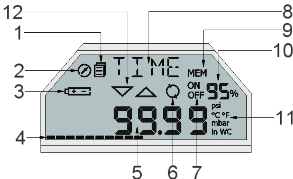
Abbildung 3: ESS3 Displayanzeigen
