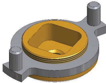
Bild 4 Bajonettadapter Art.Nr. 01301199999
